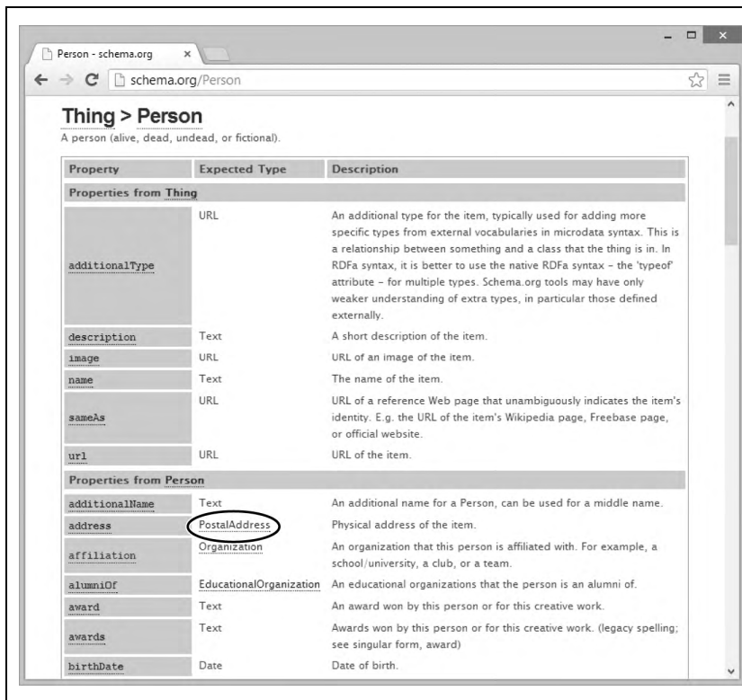
图3-5: Person词汇表的属性很多(图中只显示了一少部分)。大多数属性用于标注普通文本、数值或日期。但有一些(如这里能看到的address属性)会使用自己的词汇表(PostalAddress)。单击相应链接,可以了解更多内容
